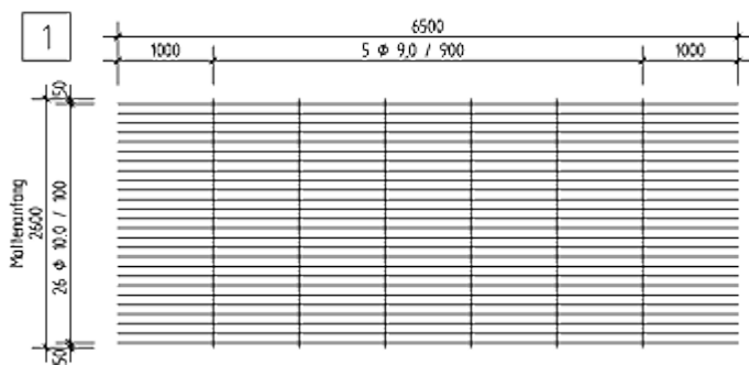
1-achs-Matte mit gleichbleibender Längs- und Querteilung
